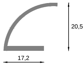
Perfil jalador
