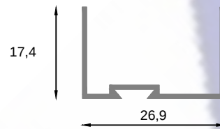
Jamba celosía (vitroven)
